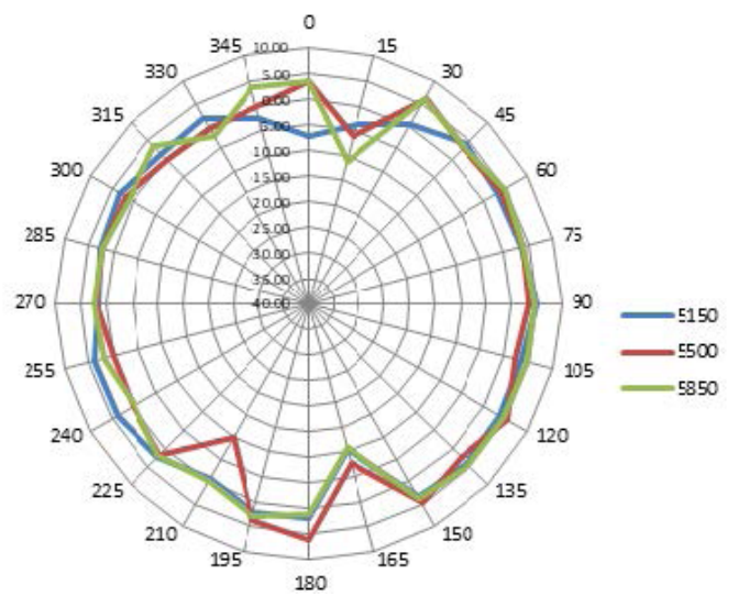
5 GHz: H-Plane
