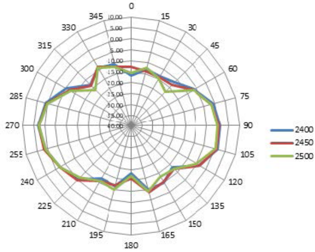
2.4 GHz: E-Plane
