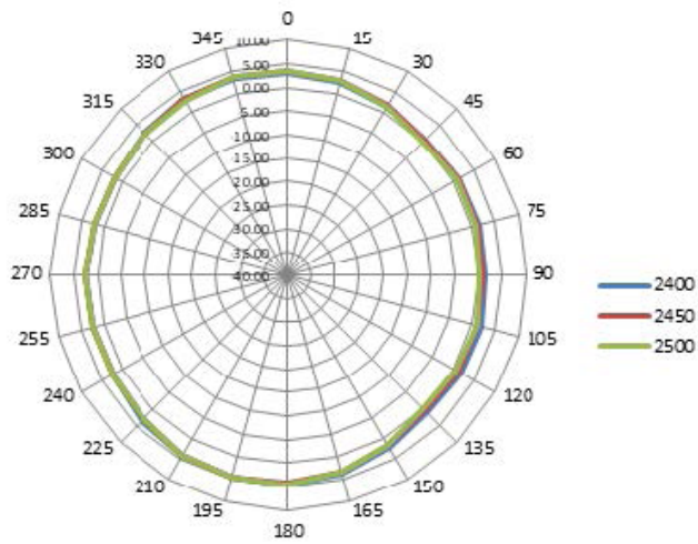
2.4 GHz: H-Plane
