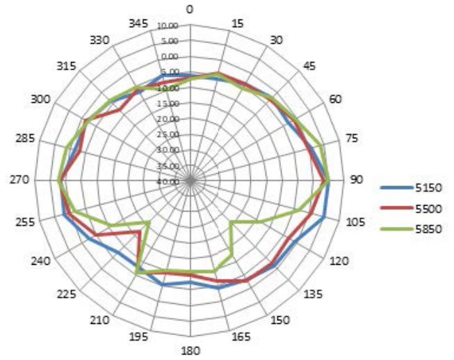
5 GHz: H-Plane
